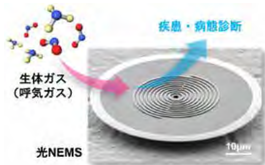
ヘルスケア（呼吸診断）用 NEMS ガスセンサデバイス NEMS gas sensing device for the healthcare (Breath diagnosis)
