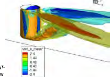
スパー型浮体式洋上風車 Spar-type floating offshore wind turbine
