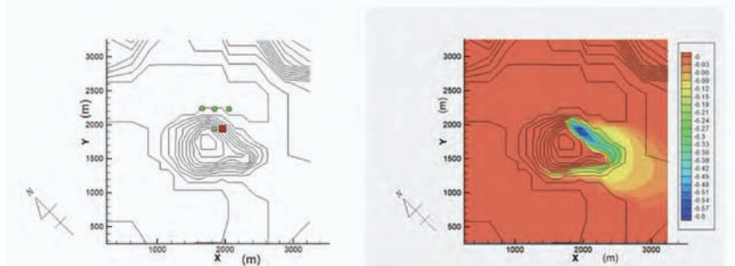
鹿児島湾内のCO 2 自然漏出位置○を観測点□から数値的に推測した確率分布
